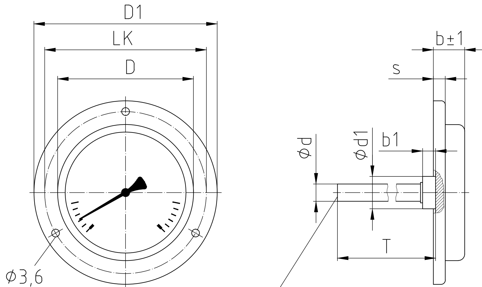
Justierschraube Schlitz
